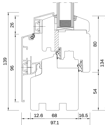
Taglio del profilo IDEALU Classicline IV 68
