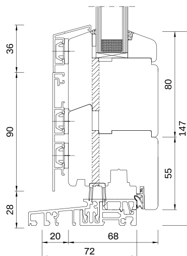
Infisso in legno-alluminio IDEALU Classicline IV 68 con soglia ribassata
