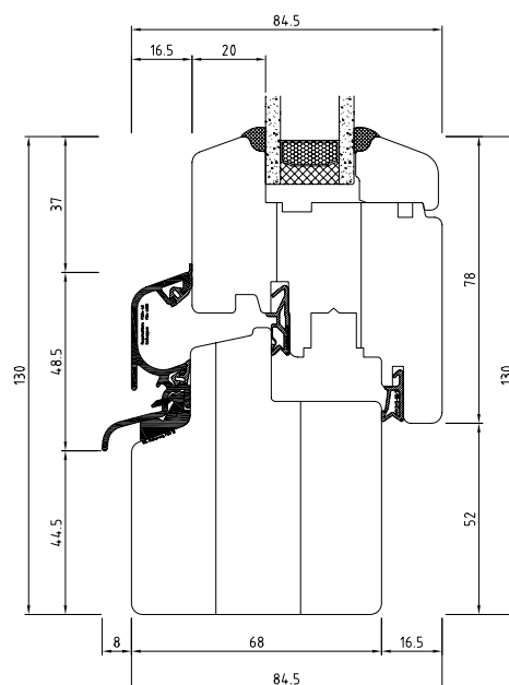
TAGLIO DEL PROFILO DELLA FINESTRA IN LEGNO CLASSICO IV 68
