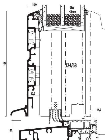
IDEALU TRENDLINE IV 68 CON SOGLIA PIATTA
