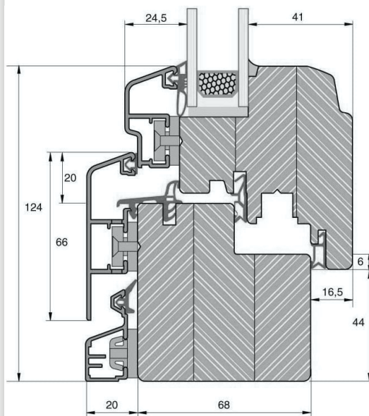
IDEALU TRENDLINE IV 68 TELAIO CON ANTA
