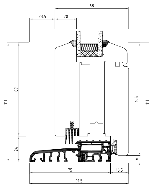
FINESTRA IN LEGNO RUSTICO IV 68 CON SOGLIA PIATTA
