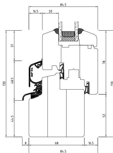
FINESTRA IN LEGNO IV 68 SEZIONE TRASVERSALE
