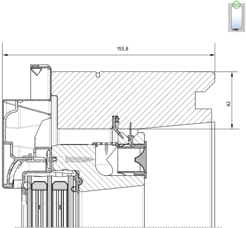
VISTA DALL'ALTO: ANTA A RIBALTA CON TRIPLO VETRO
