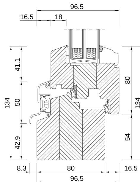
TAGLIO DEL PROFILO DELLA FINESTRA IN LEGNO RUSTICO IV 80
