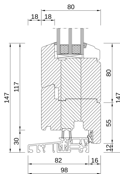
FINESTRA IN LEGNO RUSTICO IV 80 CON SOGLIA PIATTA
